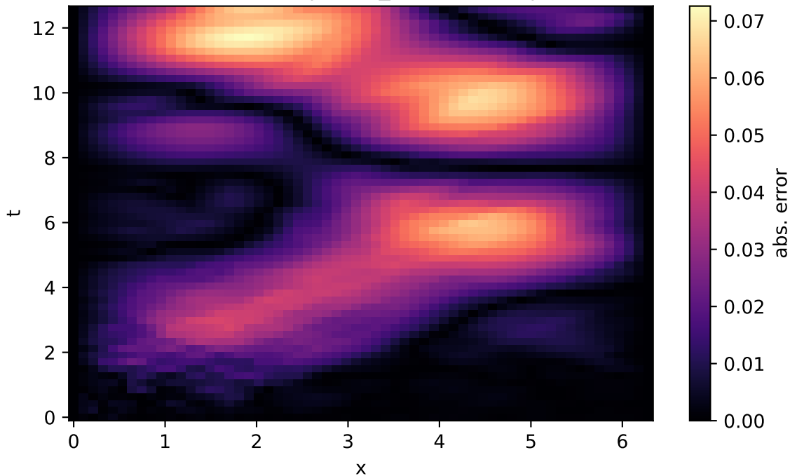
1D Wave - |KANN_cheb - exact|
