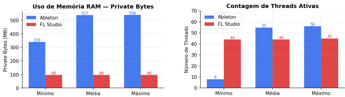
Figura 2 – RAM ( Private Bytes ) e threads em repouso — Teste 1.
