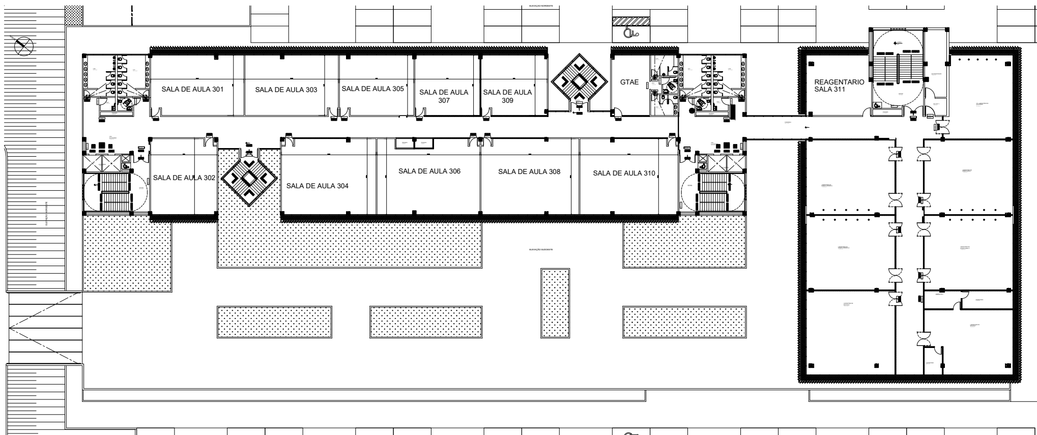
PLANTA 3º PAVIMENTO ESCALA 1:50
