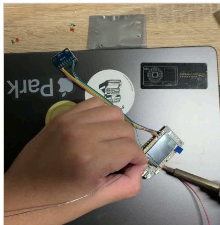
⑥ 全部焊好：主板一排線—ADXL345，蜂鳴器另一組兩芯線。
