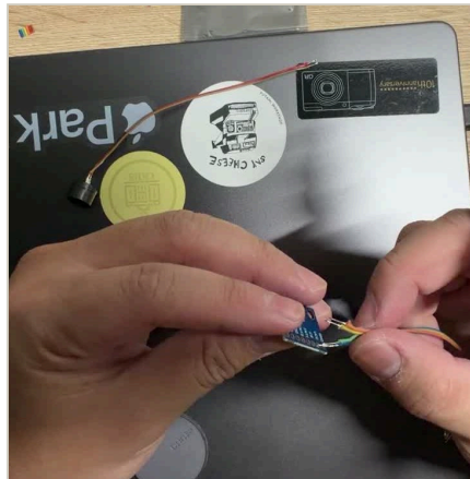
④ ADXL345：四條線穿過 VCC / GND / SDA / SCL 的通孔從背面焊，其他四孔空著。
