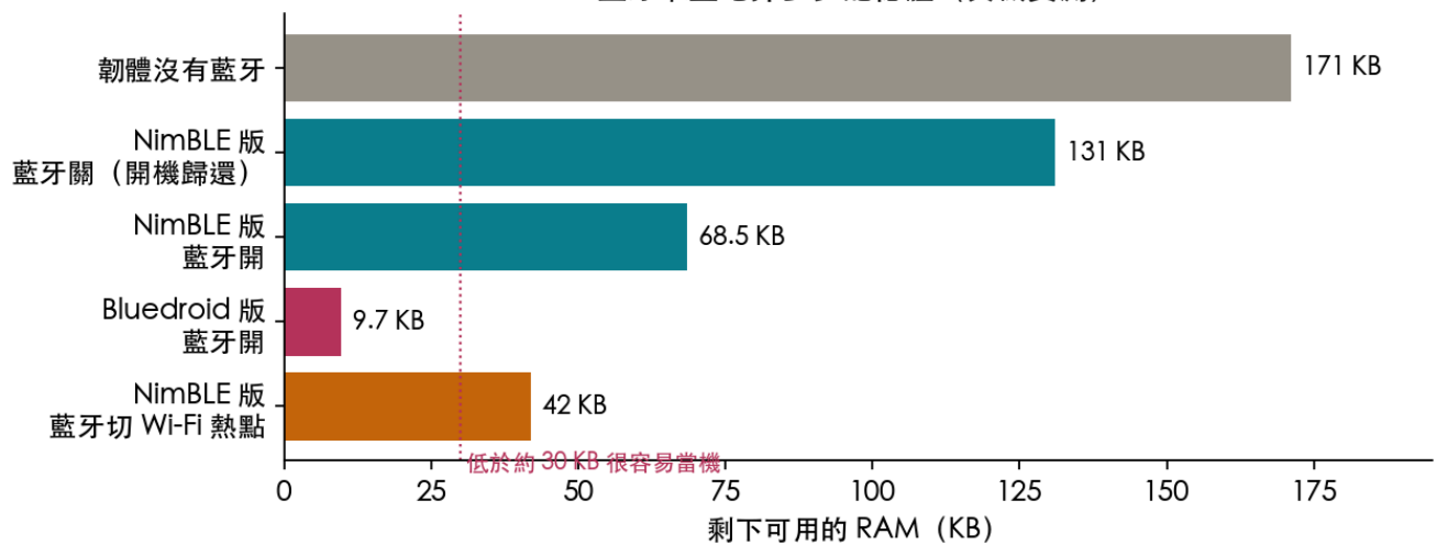
藍牙堆疊吃掉多少記憶體（真機實測）
