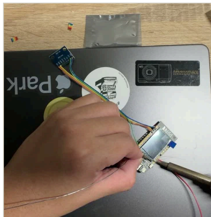
⑥ 全部焊好：主board一排線—ADXL345，蜂鳴器另一組兩芯線。
