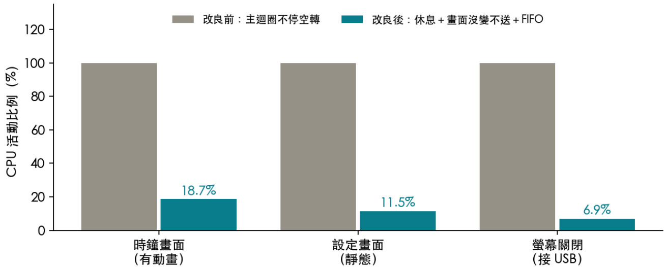
CPU 真正在做事的時間比例（真機 perf 實測）
