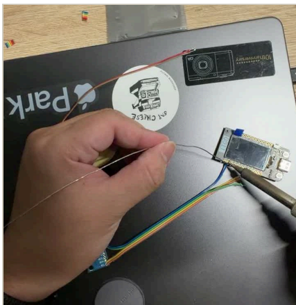
⑤ 主board端：3V、G、21、22 與 25、G 共六孔，排針孔比模組大，容易焊。
