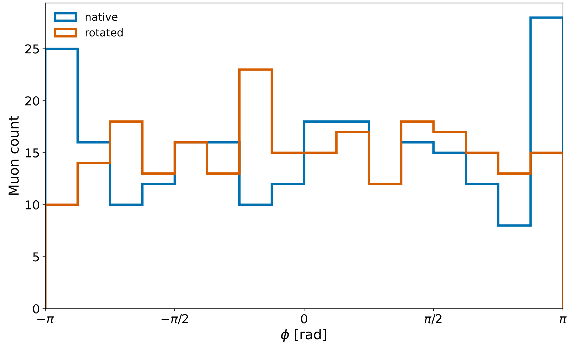
Muon momentum \phi ( E < 1 GeV)
