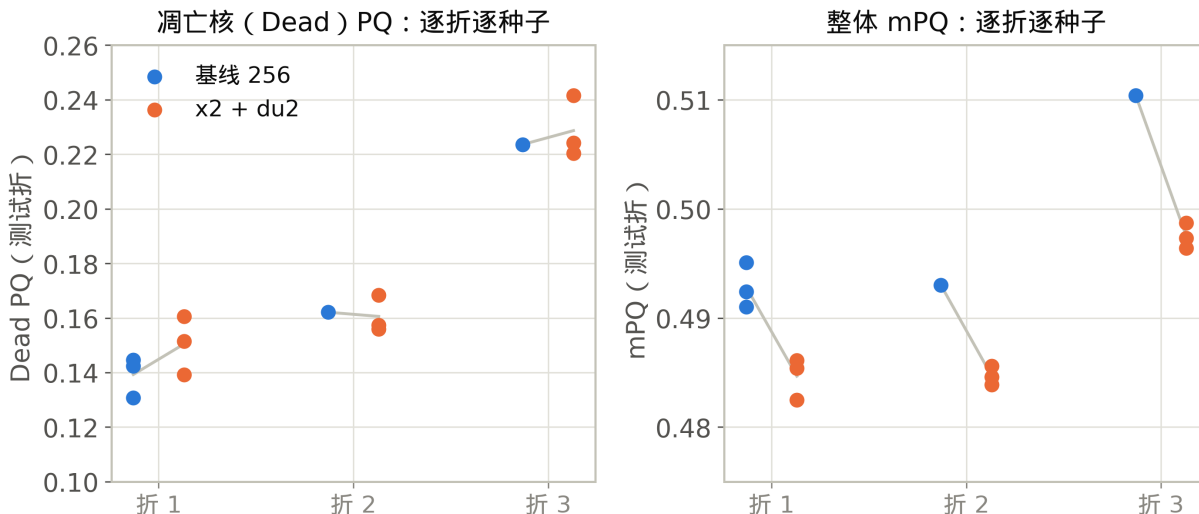
图 4: 种子网格。右: mPQ——每个分裂上全部 du2 run (橙) 都低于基线 run (蓝), 代价毫无歧义。左: Dead PQ——run 相互交错; 分裂 2 的 du2 种子均值落在基线种子之下, 分裂 3 的种子 19 翻号。连线为种子均值 (基线额外种子只在分裂 1 存在)。
