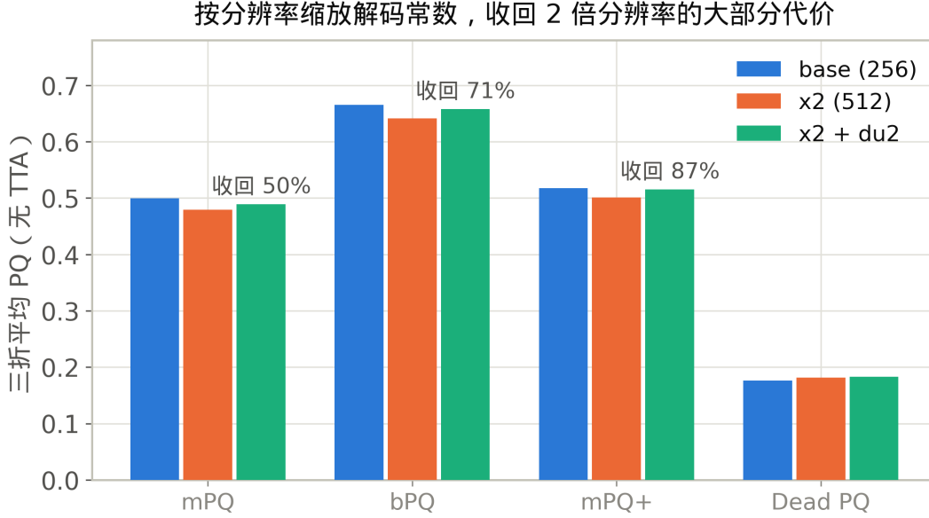
图 3: 表 3 (无 TTA): 缩放两个解码常数即收回 2× 聚合代价的大部分, 同时 Dead 增益存活; mPQ + 与基线的差距缩到.002 以内。
