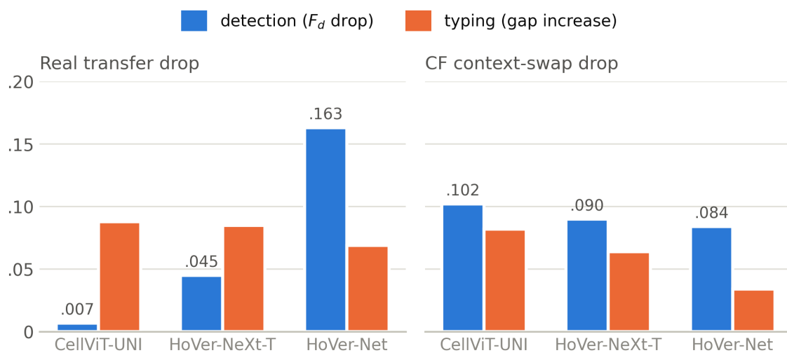
图 6: 轴分解 (架构均值; 表 6): 真实迁移的架构差异集中在检测轴 (左图 F_d 降幅), 而 CF 上下文交换压力对检测的影响在架构间齐平、只对分型轴携带排序信息 (右图)。
