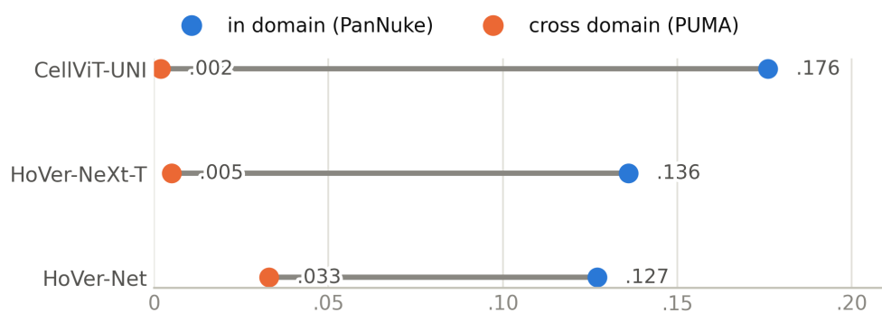
图 4: 各架构的 Dead PQ: 域内 (PanNuke, 3-split 均值) 与 PUMA 零样本跨域对比。该类随模型跨域几乎归零 (0.002–0.033, 域内为 0.127–0.176)。
