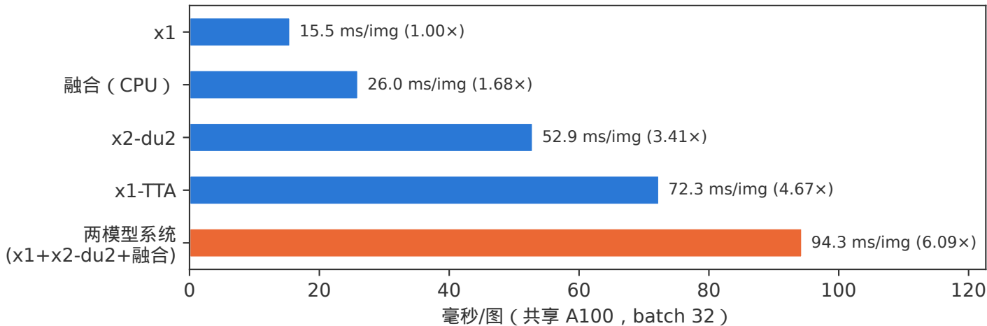
E0 推理成本：EF-P2 两模型系统 vs 单模型 x1
