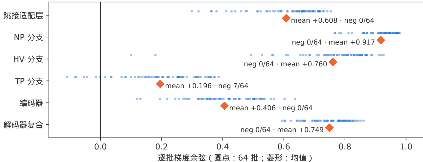
DSB 闸门 B 修正重跑：Dead 与常见类梯度 ( fold 1 )
