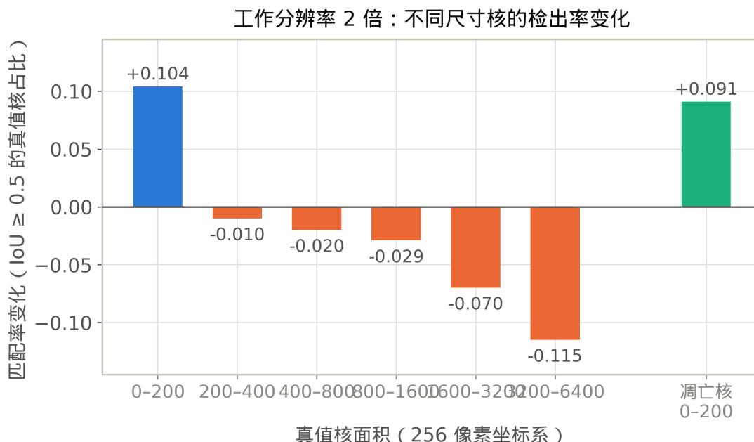
图 1: 2× 分辨率带来的匹配率变化, 按真值核面积分层 (分裂 1 TTA, x2 种子 19 减 3 种子基线均值; IoU ≥ 0.5)。效应是尺寸的单调函数, 与类别无关: 200 px 以下的核全部获益 (含 Dead, +.091), 400 px 以上的尺寸段全部受损, 单调递减。每个尺寸段内匹配对的 IoU 持平 (±.01)。
