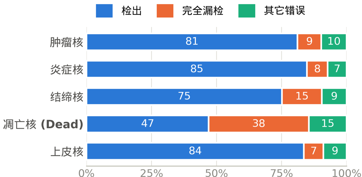
图 1: 五类细胞核的错误分解 (CellViT-UNI, 折 3)。蓝色“检出”指预测轮廓与人工标注重叠过半; 橙色“完全漏检”指模型答案里根本没有这个核。凋亡核 (Dead) 一行有 38% 完全漏检, 是其它类的 3-5 倍。
