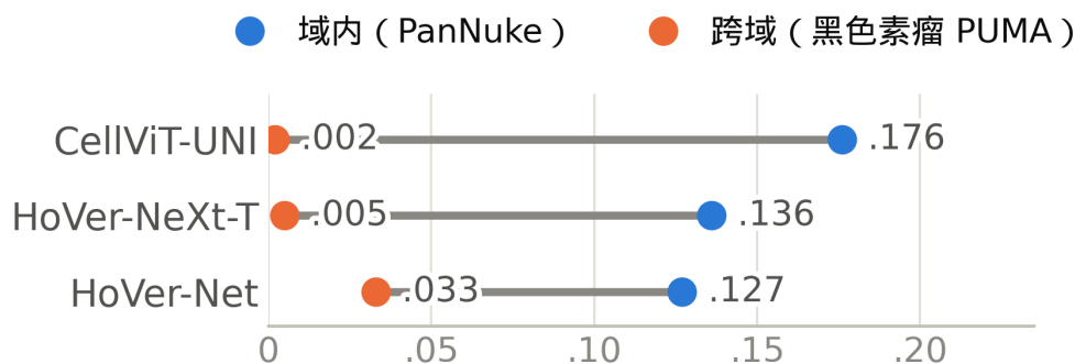
图 3: 三种模型的凋亡核 (Dead) 得分: 域内考试 (PanNuke) vs. 跨域考试 (黑色素瘤数据 PUMA)。跨域时所有模型的凋亡核得分都跌到接近 0。
