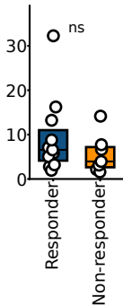
CD4_T
