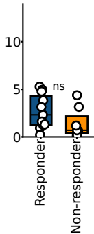
Stromal
