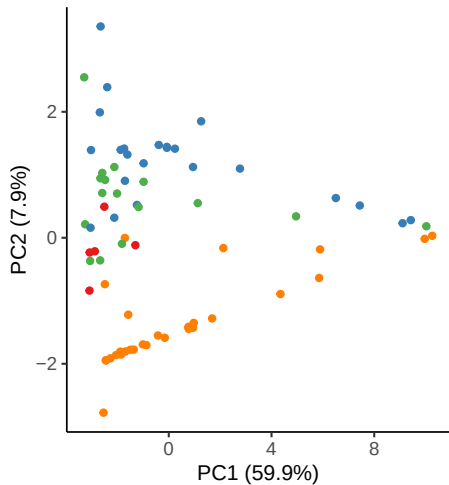
Deconvolution PCA
