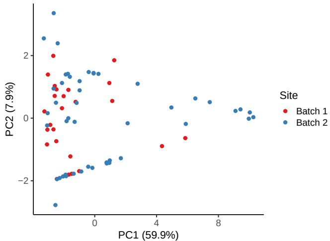
Deconvolution PCA
