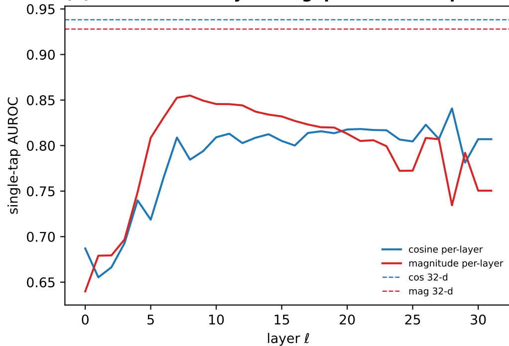
(d) H9d redundancy: 32-d gap over best tap
