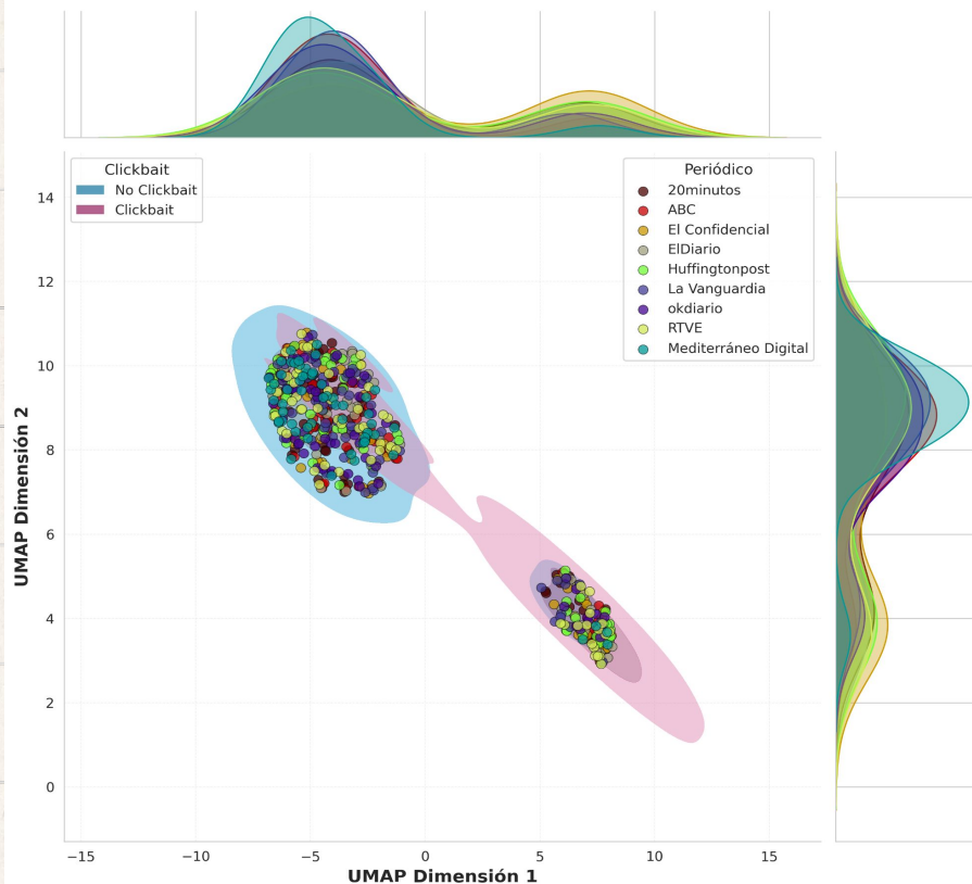
Espacios Embebidos de Títulos por Periódico - Análisis UMAP
