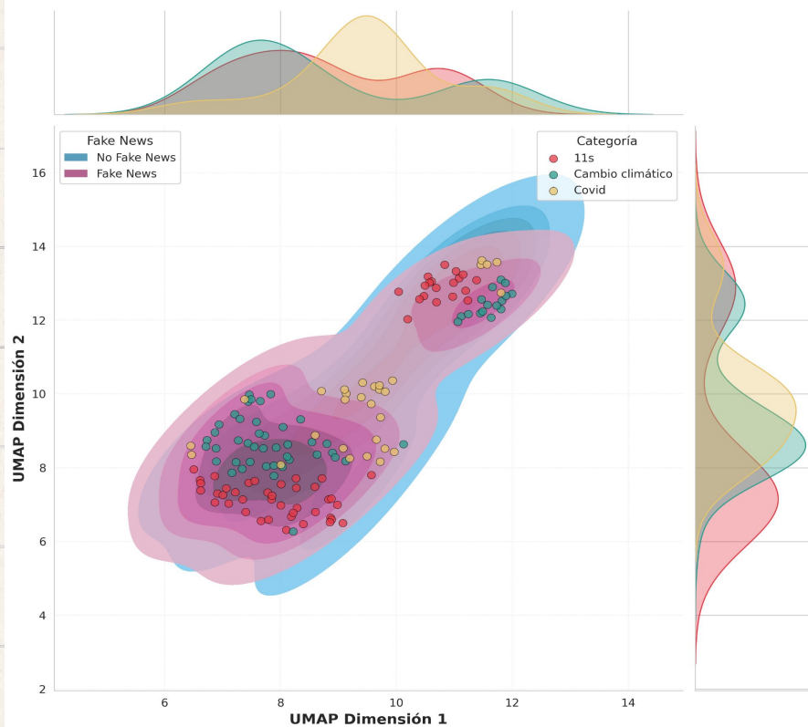
Espacios Embebidos de Títulos - UMAP
