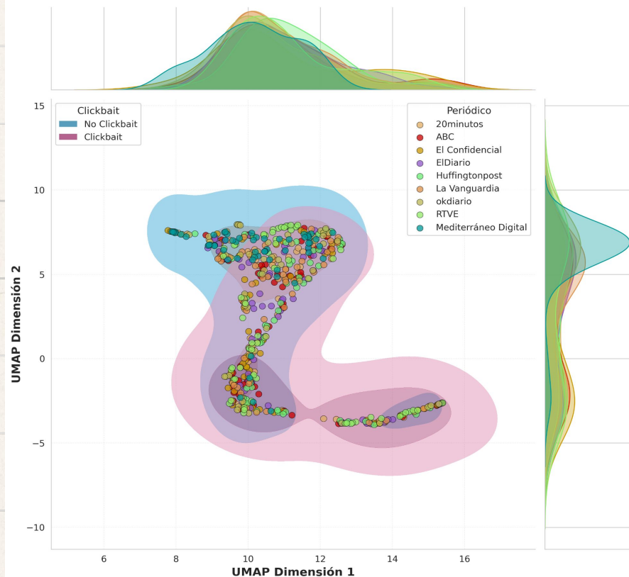
Espacios Embebidos de Contenido por Periódico - Análisis UMAP
