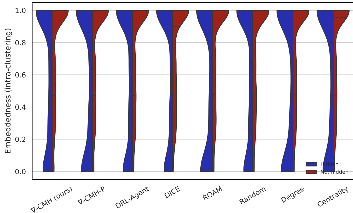
cond-mat — leiden
