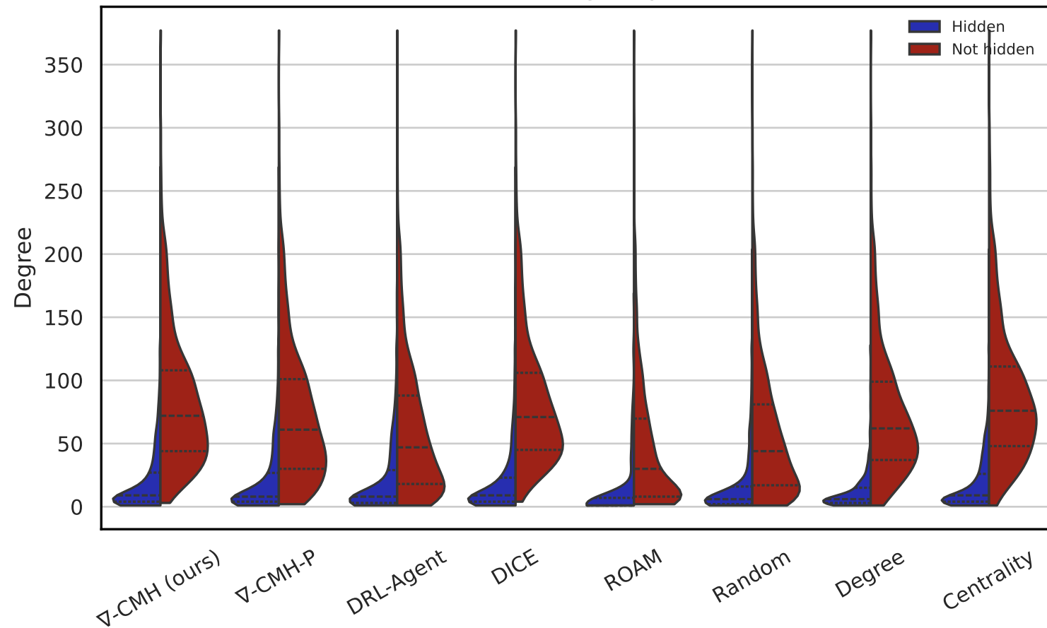
fb-75 — greedy
