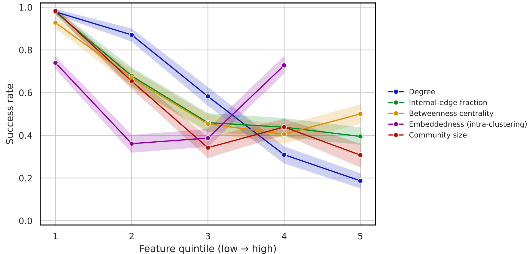
fb-75 — walktrap — \nabla -CMH
