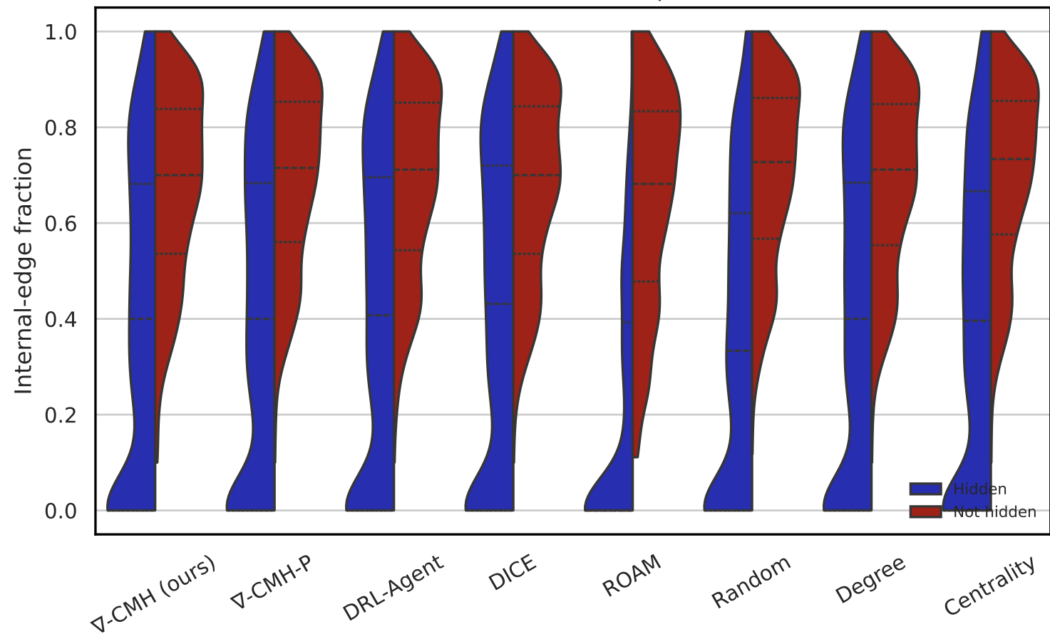
fb-75 — walktrap
