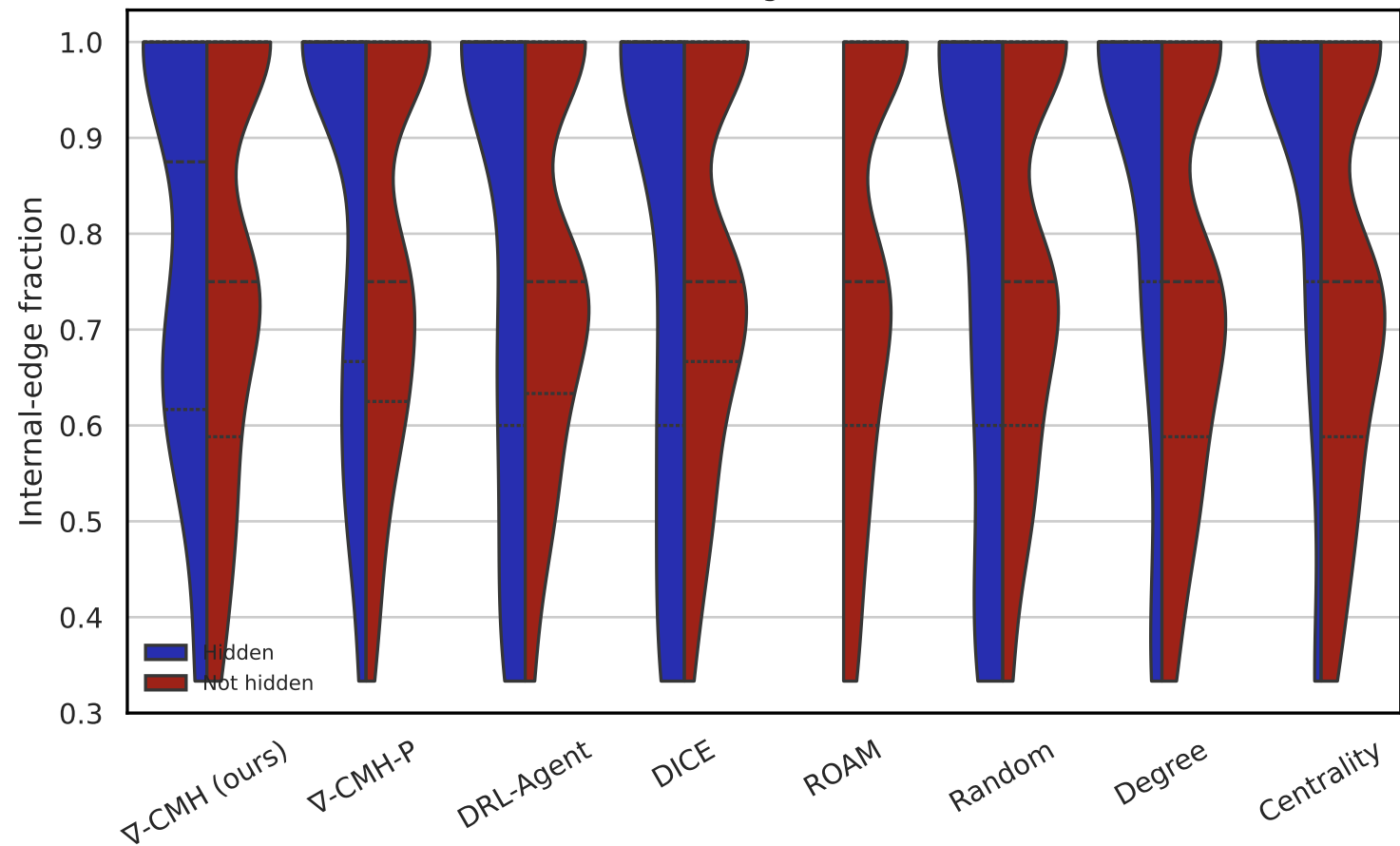
kar — dgcluster
