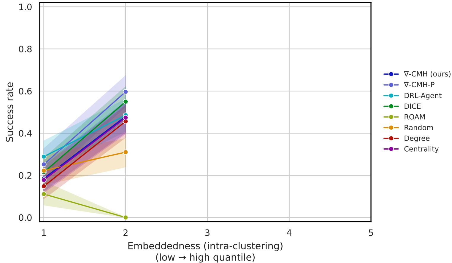
kar — leiden
