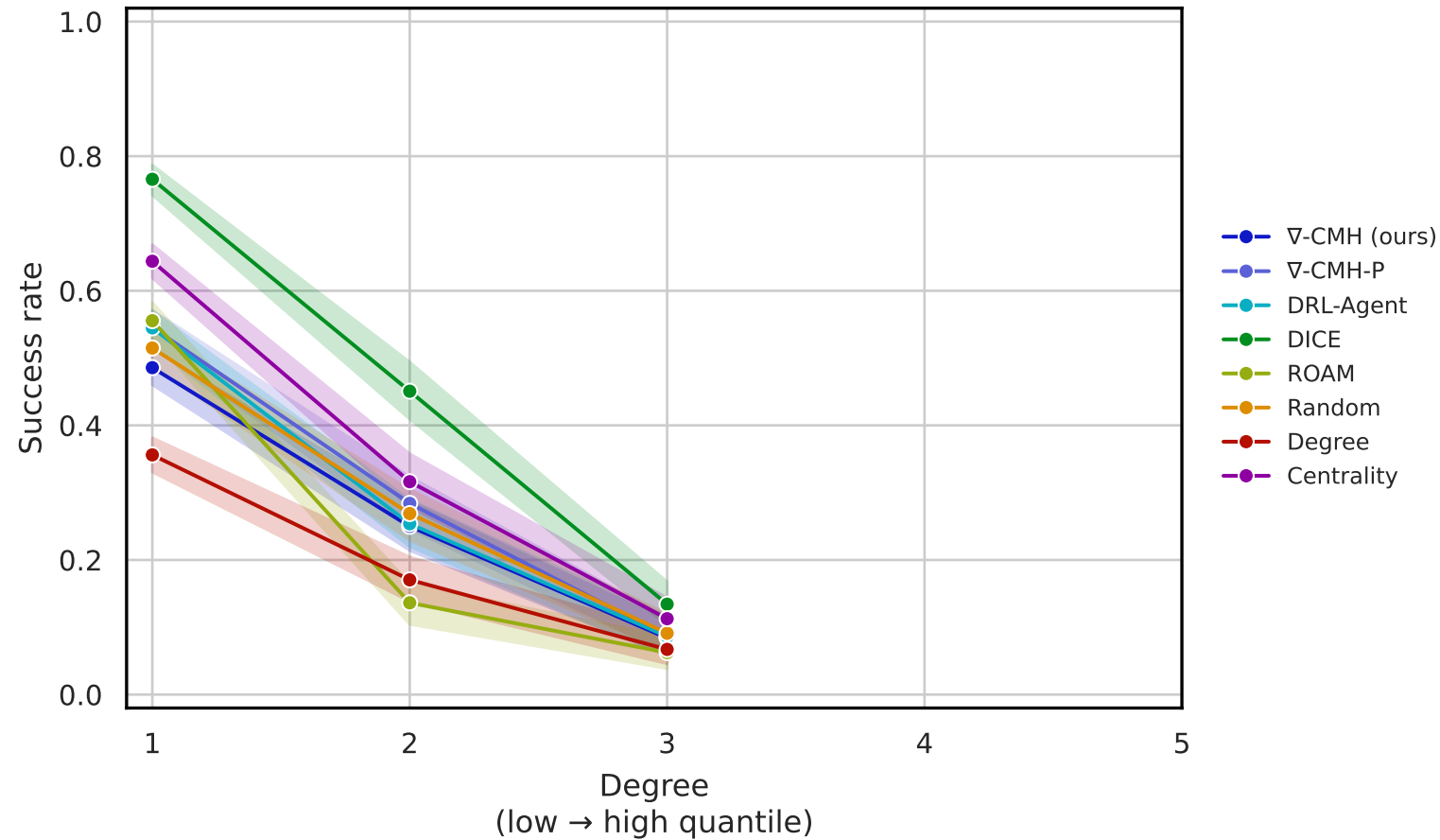
pow — leiden
