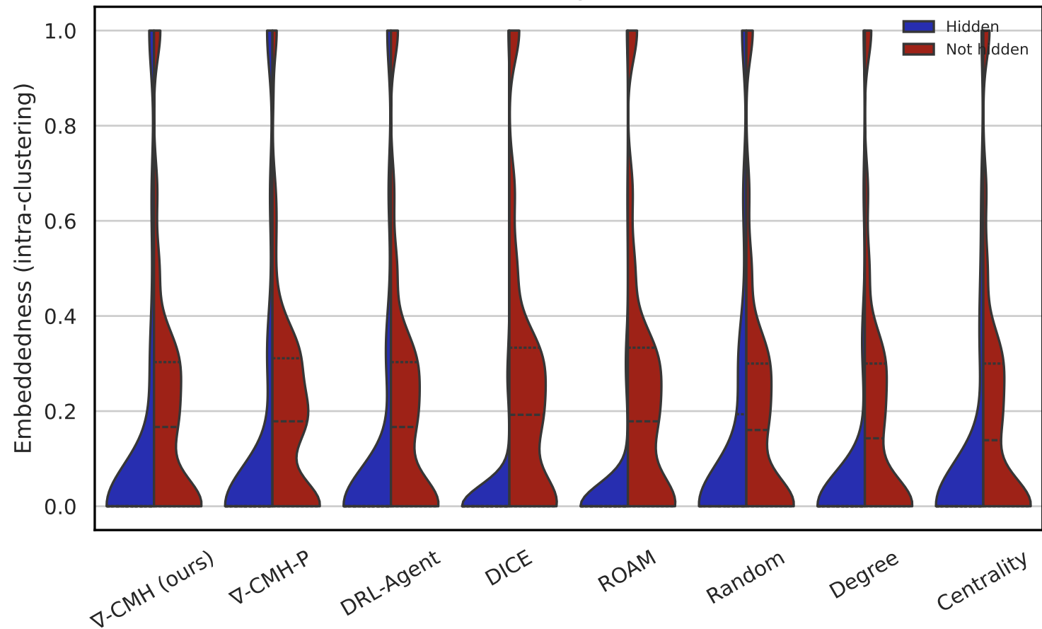
vote — dgcluster
