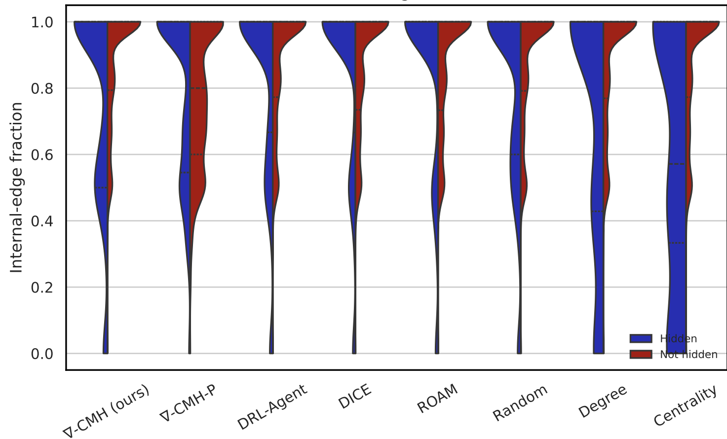
vote — dgcluster
