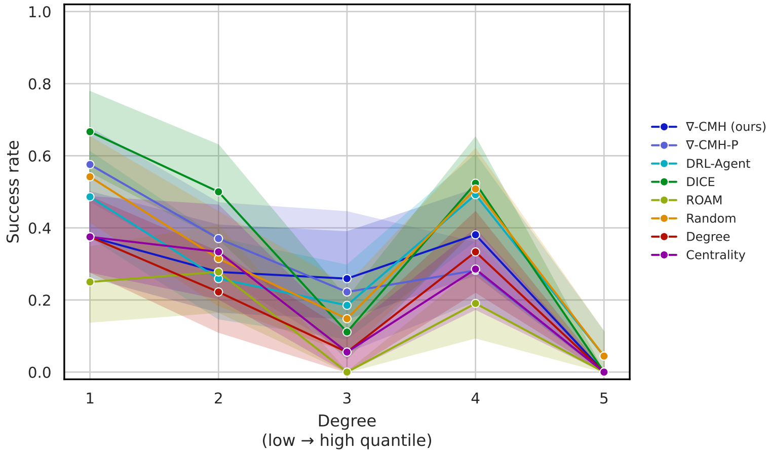
words — dgcluster
