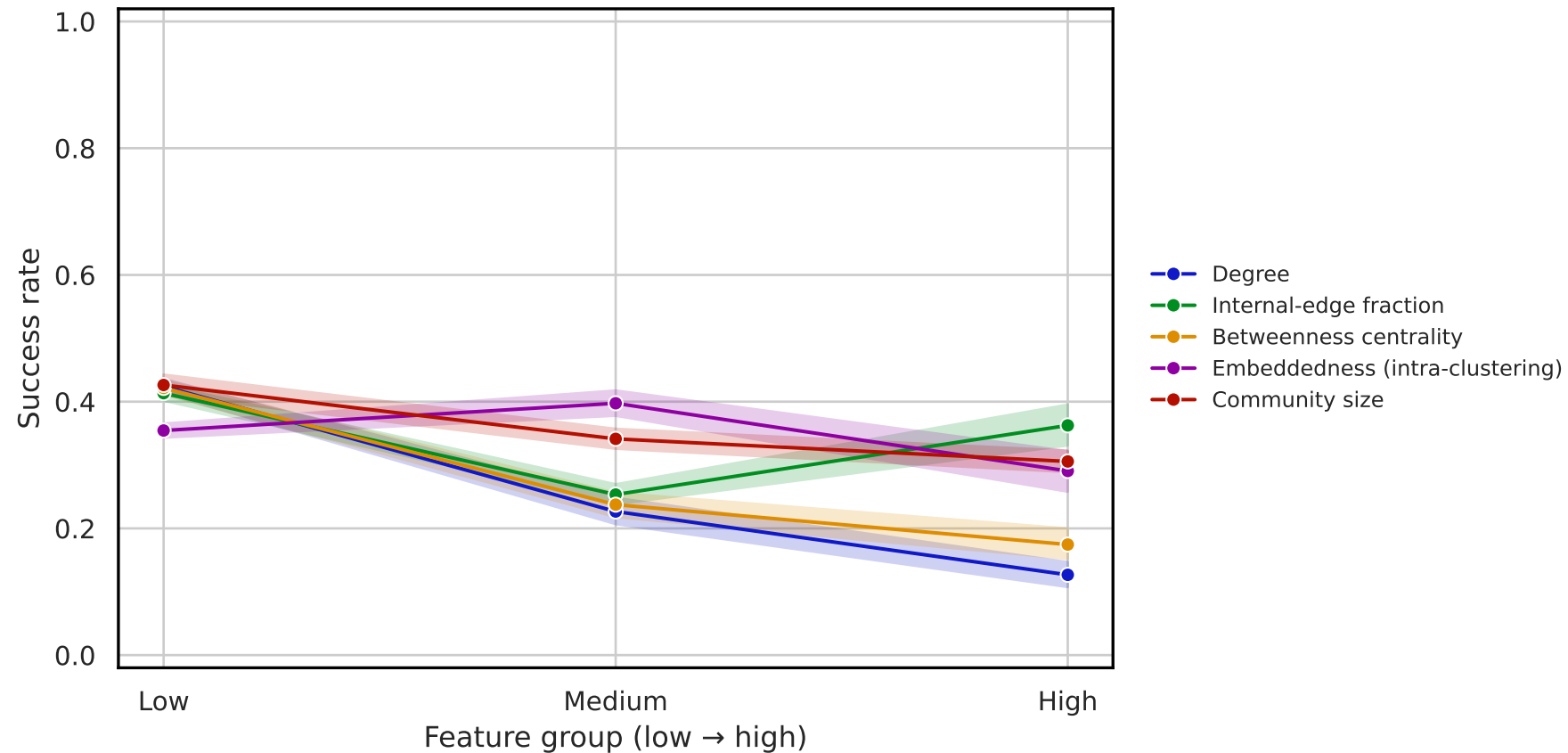
all datasets — dgcluster — \nabla -CMH
