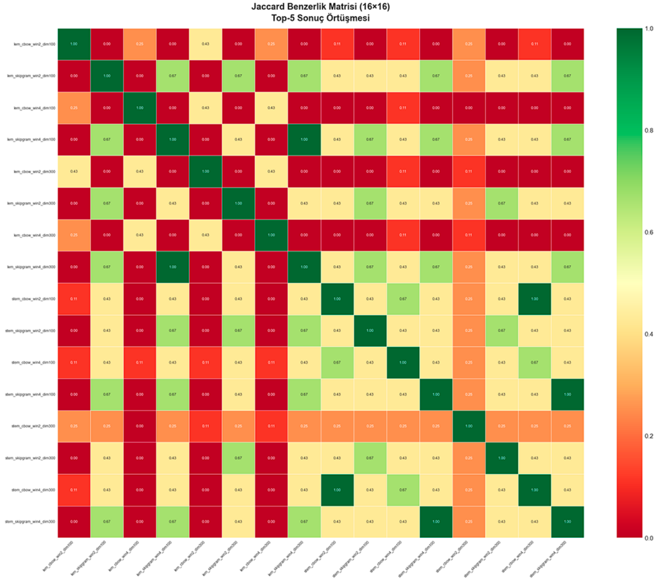
Şekil 1: Jaccard Benzerlik Matrisi Heatmap (16×16) — Modellerin Top-5 Sonuç Ortusme Oranı. Kosegen her zaman 1.00'dir (modelin kendisiyle karşılaştırması); yorumlamada hesaba katılmaz.
