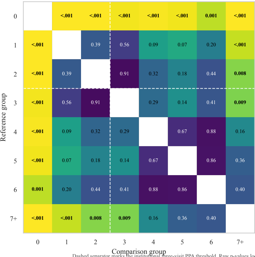
Raw pairwise p-values
