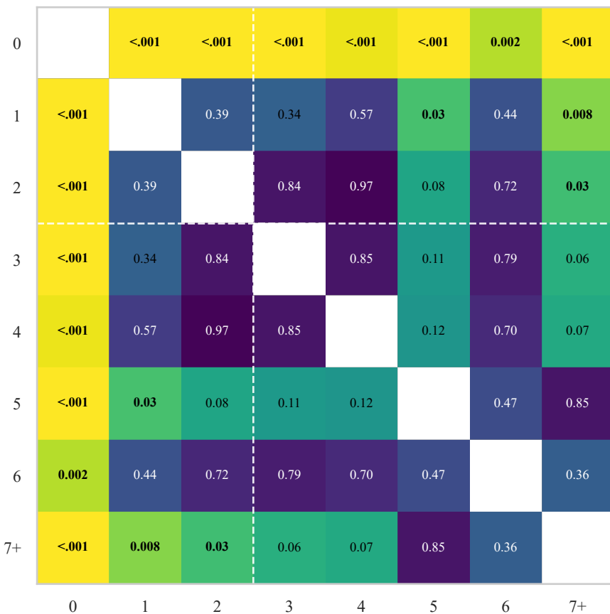
Raw pairwise p-values
