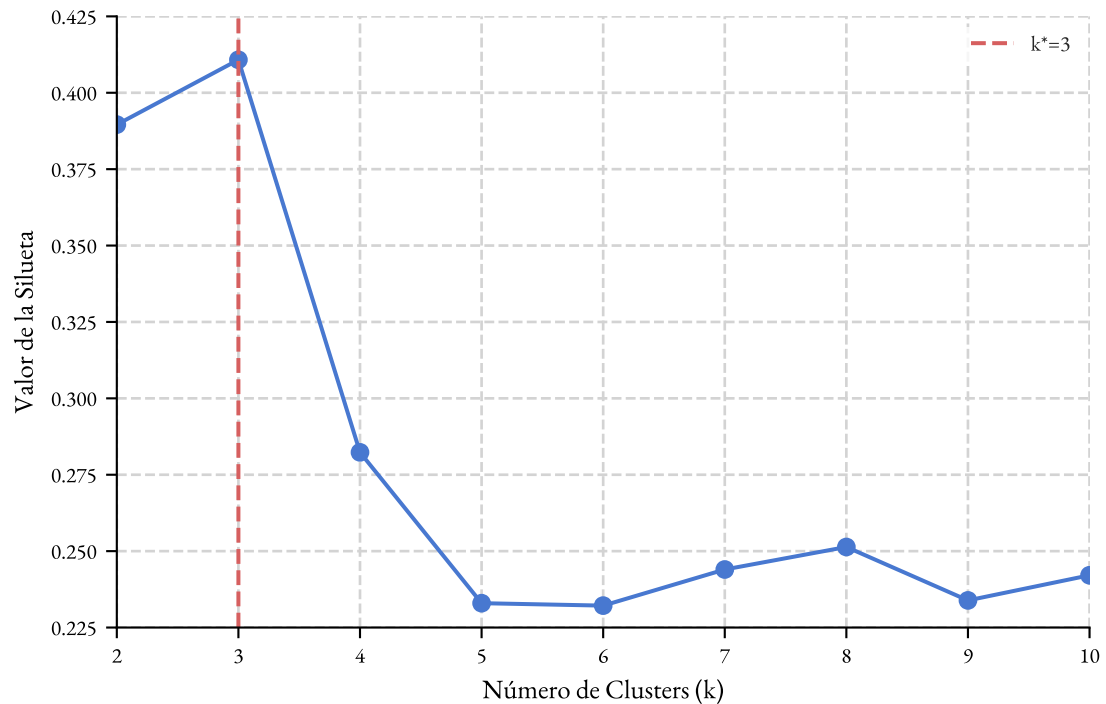
Valor de la Silueta para K-Medoids Clustering
