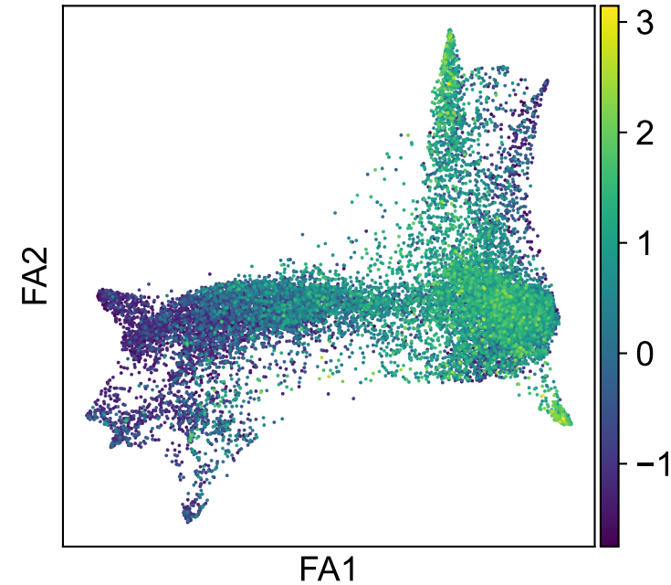
Slc35f1
