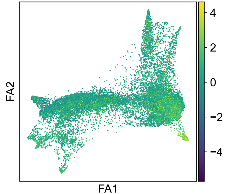
Ankrd44
