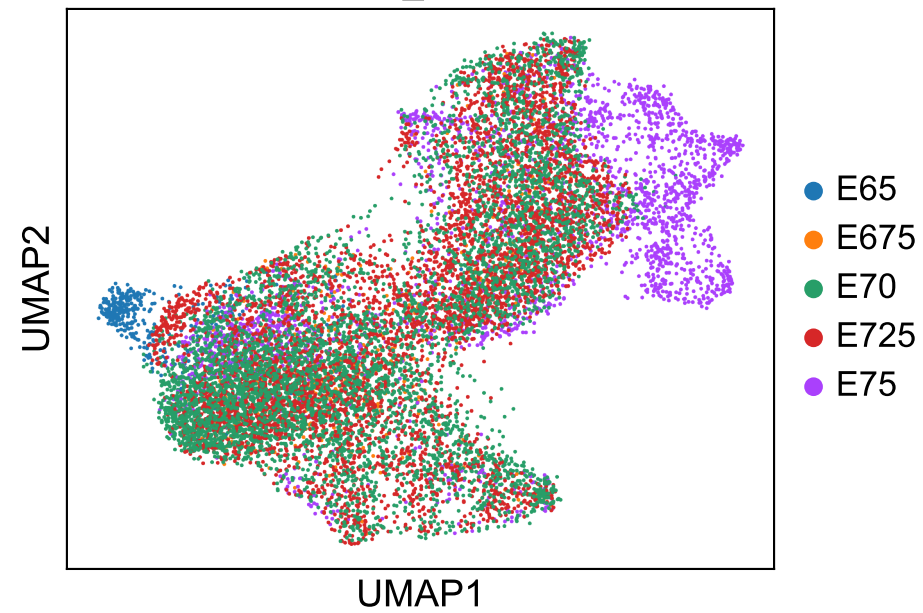
cell_time
