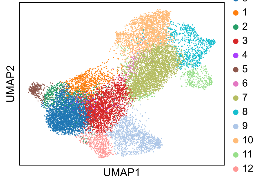
leiden
