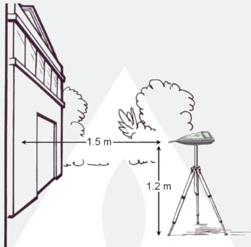
Figura. Ubicación del sonómetro según Resolución 0627 de 2006
