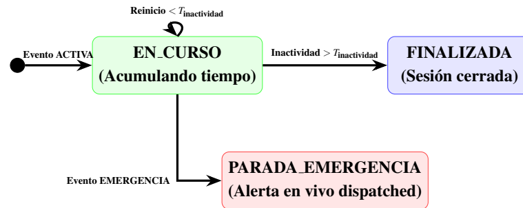
Figura 2. Diagrama de estados de la lógica de consolidación de actividades.
