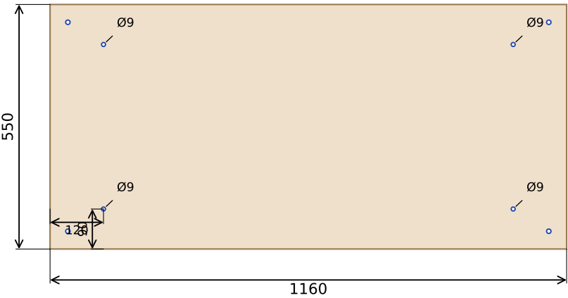
S2 · BATENTE LAT. · 2 peças
