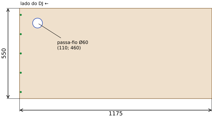
K · TAMPO DE TRABALHO · 1 peça
