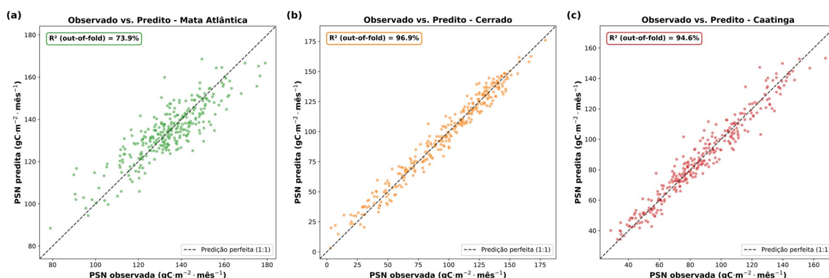
Figura 6 - Observado vs. predito do MRMP-N nos três biomas.
