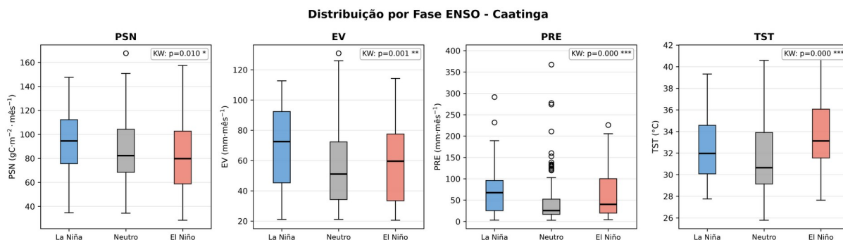
Figura 13 - Distribuição das variáveis ambientais por fase ENSO na Caatinga.
