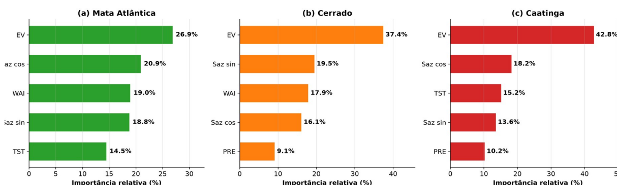
Figura 8 - Importância relativa das variáveis preditoras no modelo MRMP-N nos três biomas.
