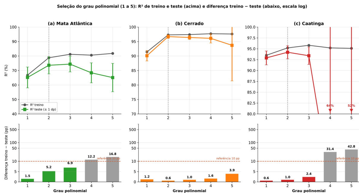
Figura 7 - Seleção do grau polinomial do MRMP-N nos três biomas: R^2 de treino e teste e diferença treino–teste por grau.
