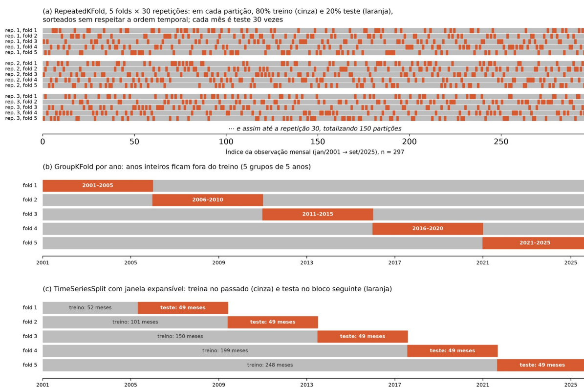
Figura 4 - Esquemas de particionamento treino/teste: (a) RepeatedKfold 5 \times 30 ; (b) GroupKfold por ano; (c) TimeSeriesSplit com janela expansível.
