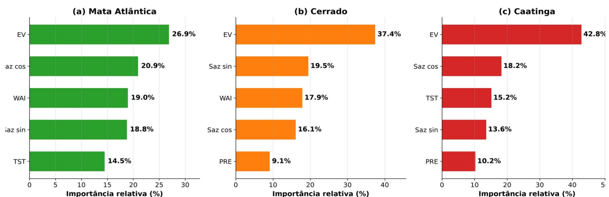
Figura 8 - Importância relativa das variáveis preditoras no modelo MRMP-N nos três biomas.
