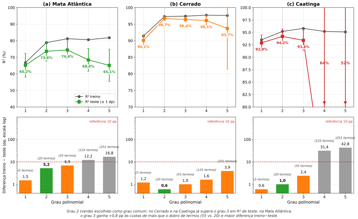
Figure 4: Seleção do grau polinomial do MRMP-N nos três biomas: R^2 de treino e de teste e diferença treino-teste por grau (RepeatedKFold 5 \times 30 ).
