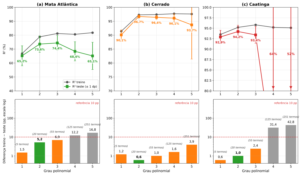
Figure 4: Seleção do grau polinomial do MRMP-N nos três biomas: R^2 de treino e de teste e diferença treino-teste por grau (RepeatedKFold 5 \times 30 ).
