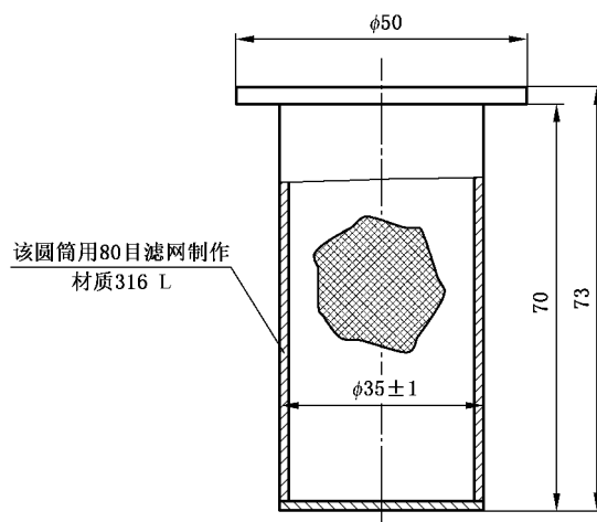
图 2 过滤网筒
