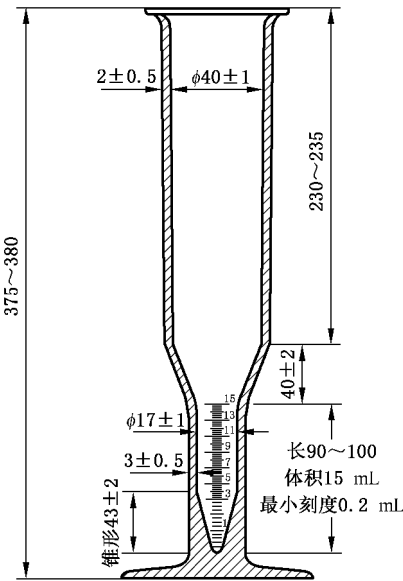
图 1 松脂油水测定器
