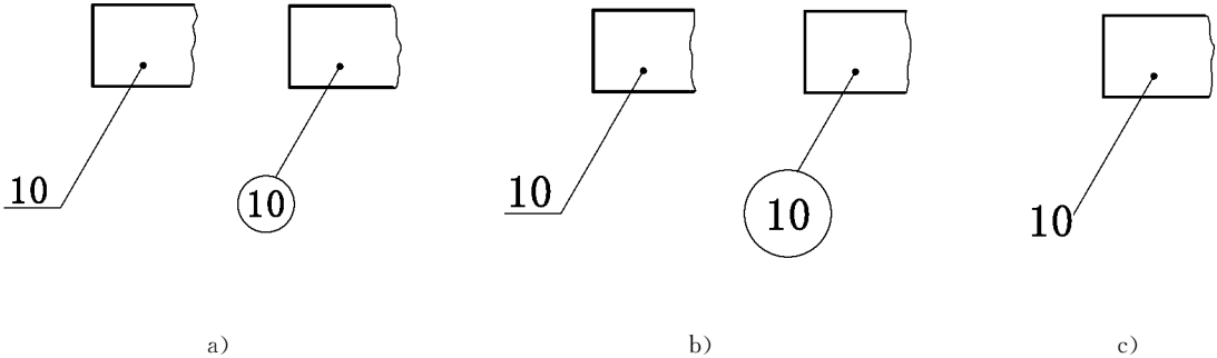
图 1 装配图中编注序号的方法
