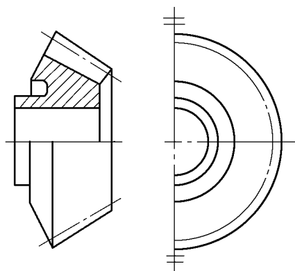
图 2 锥齿轮画法
