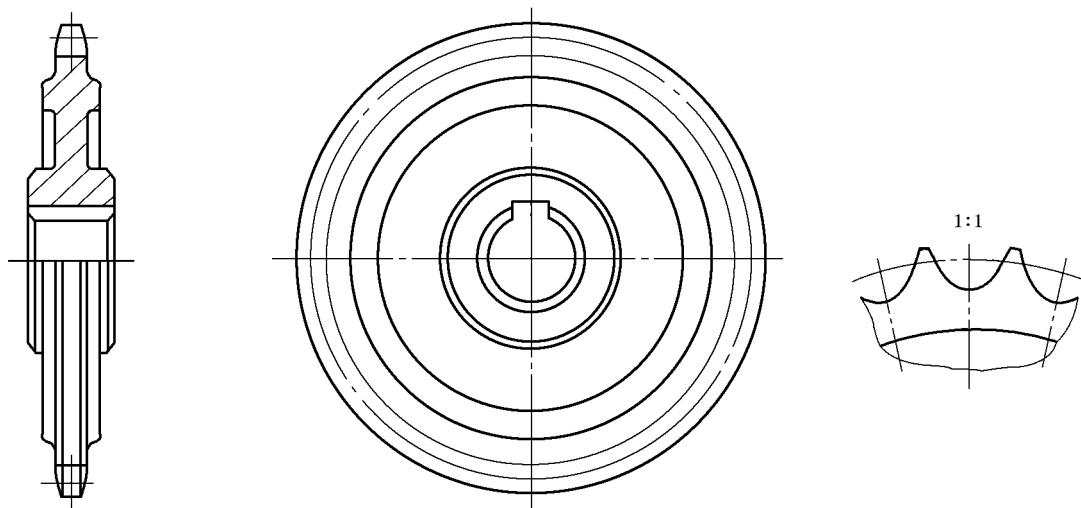
图 7 链轮画法
