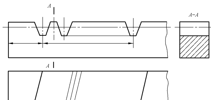
图 4 齿条画法
