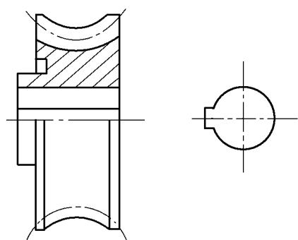
图 3 蜗轮画法
