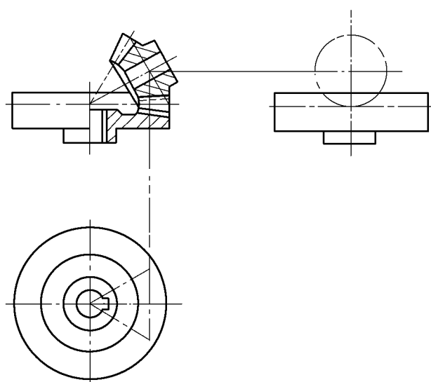
图 18 轴线斜交的平面齿轮与锥齿轮的啮合画法
