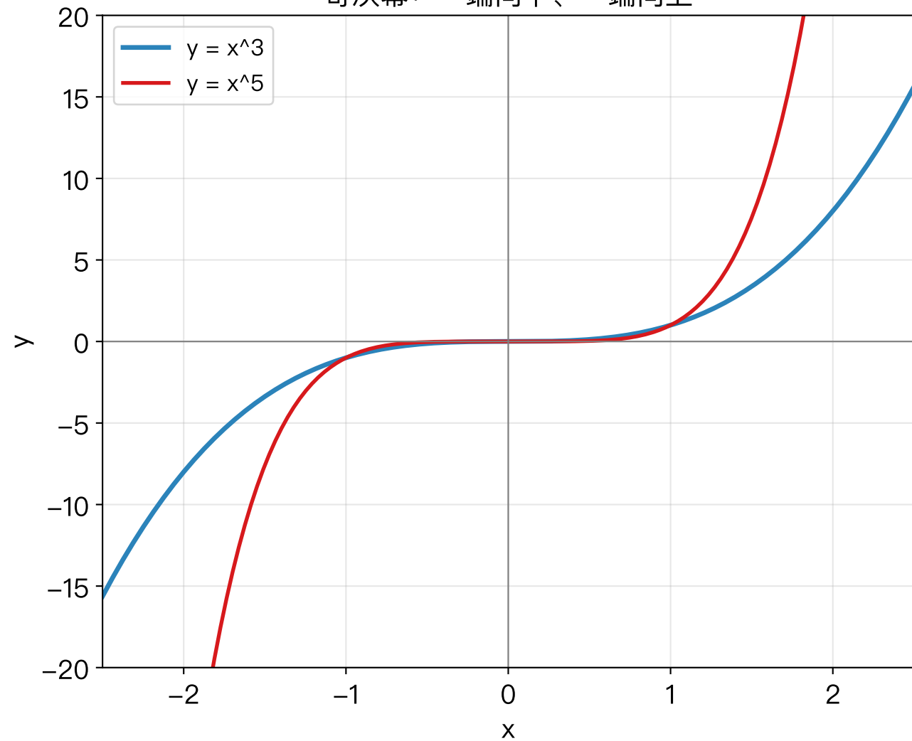
奇次幂：一端向下、一端向上
