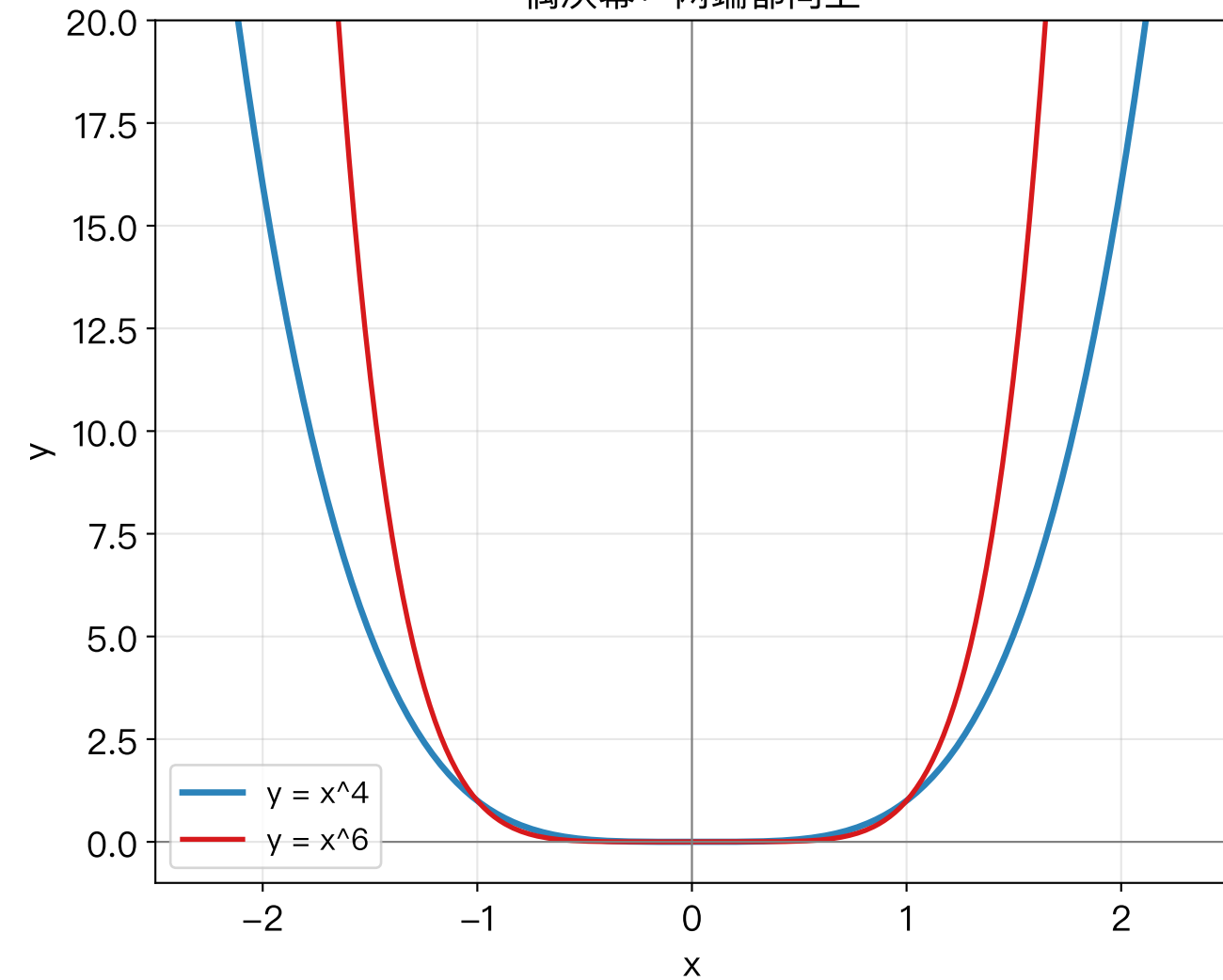
偶次幂：两端都向上
