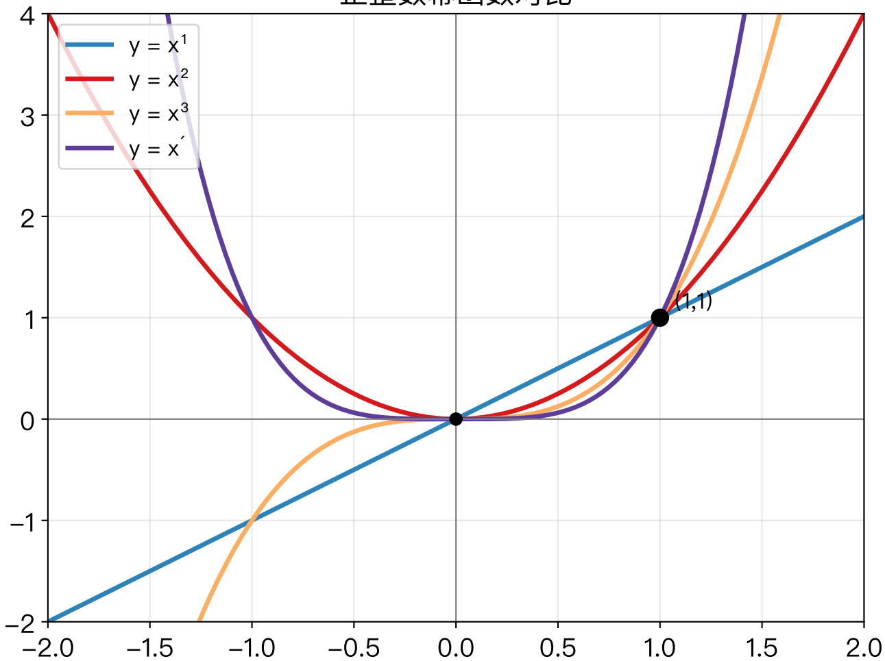
正整数幂函数对比
