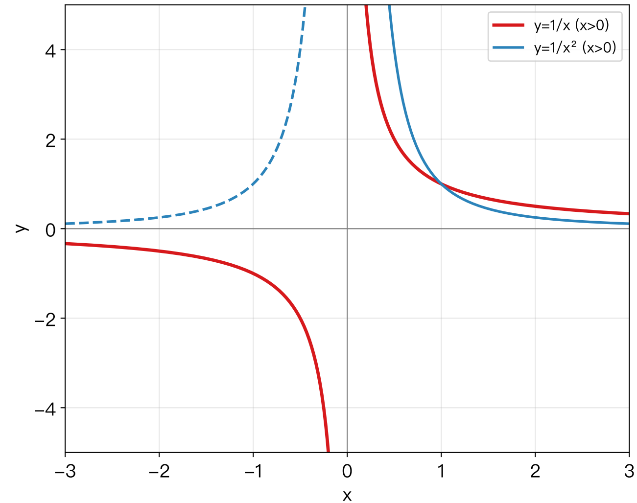
负整数幂
