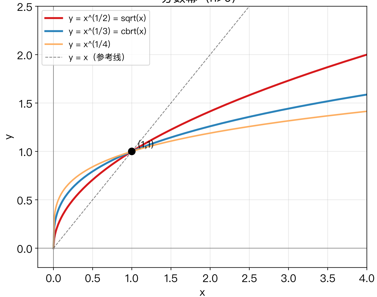
分数幂 ( n > 0 )
