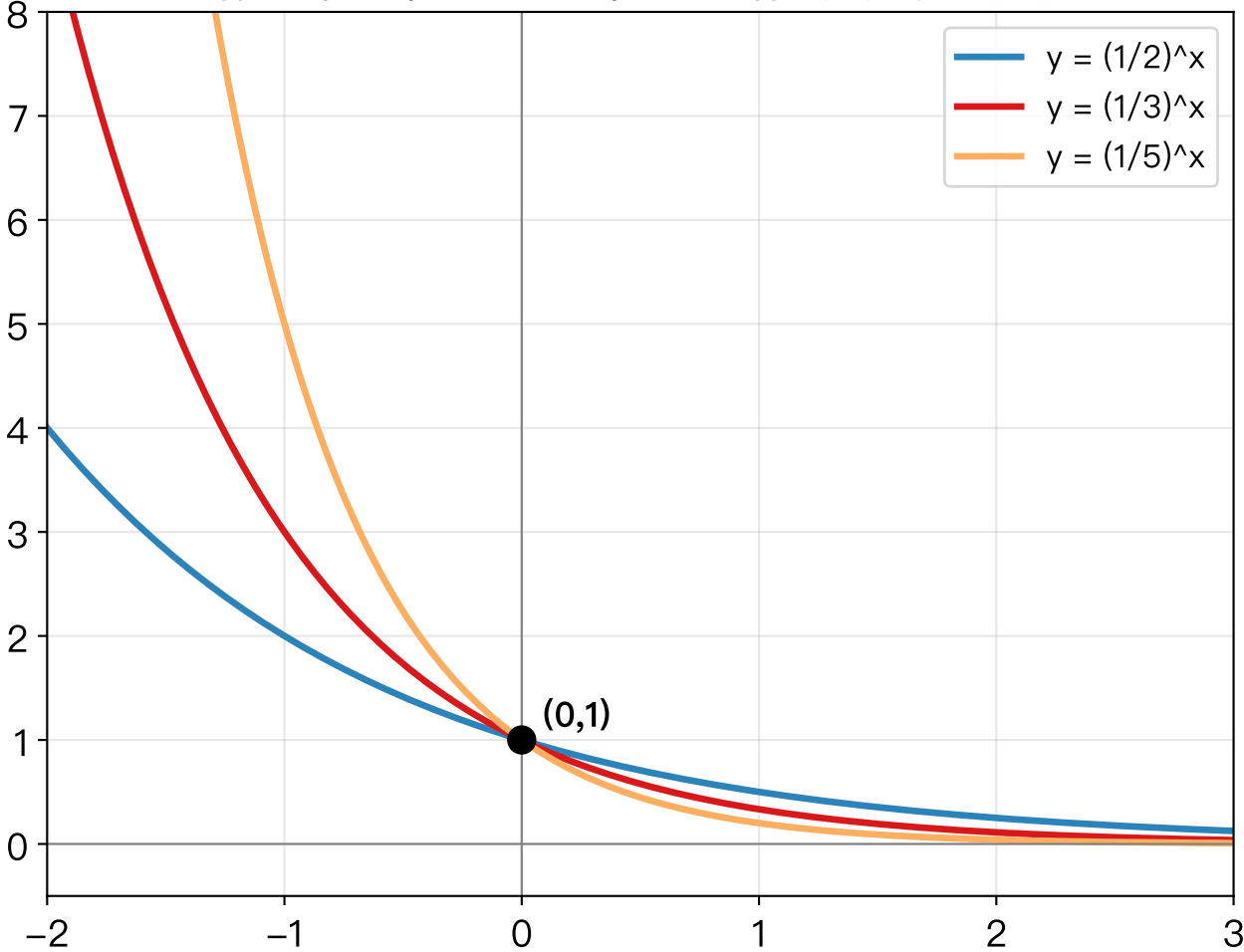
指数函数 ( 0 < \text{底} < 1 ) —— 指数越大衰减越快
