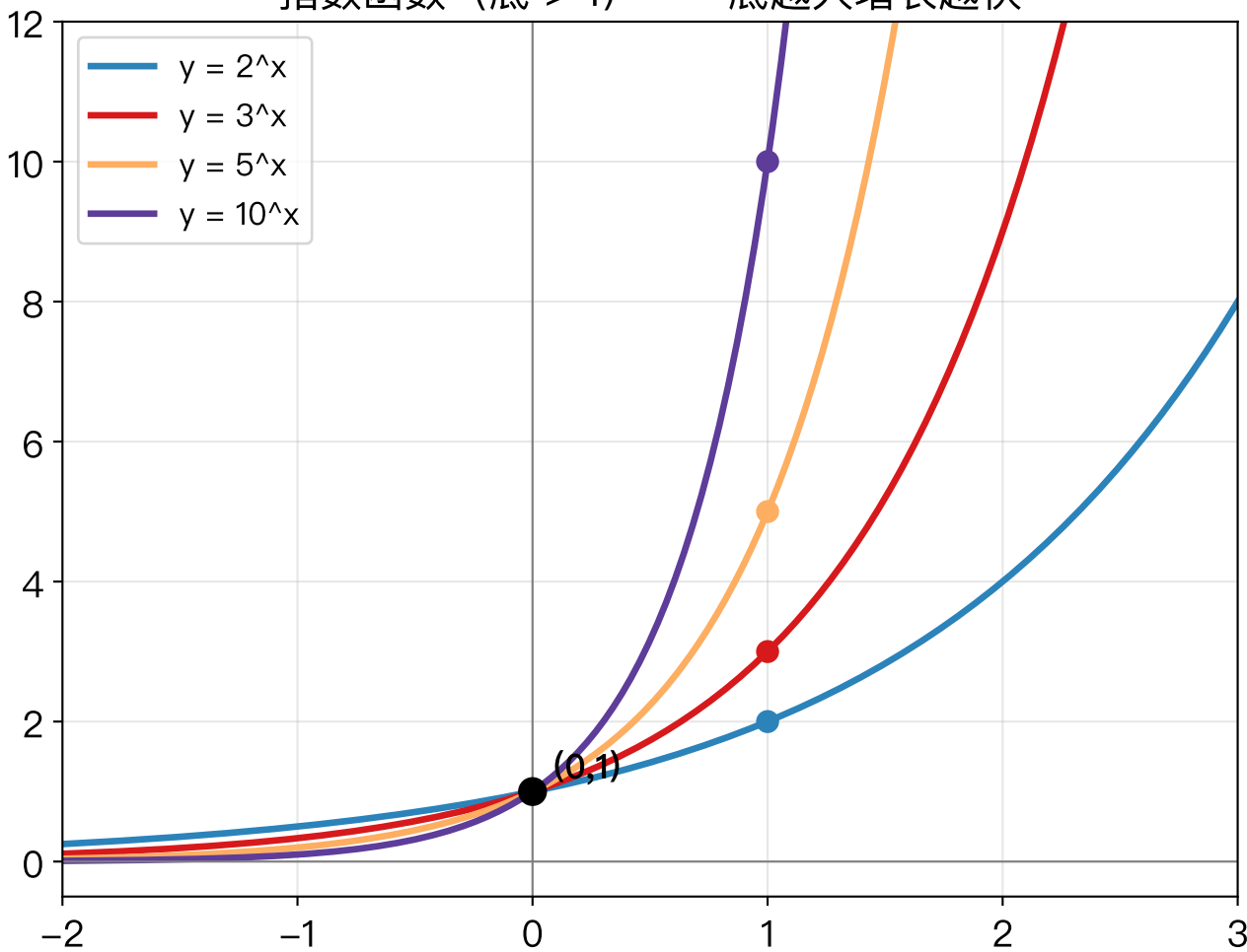
指数函数（底 > 1）——底越大增长越快
